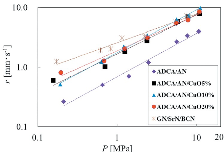
図2 ADCA/AN系ガス発生剤の線燃焼速度
